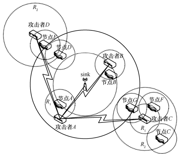
图 4 SenLeash 约束防御虫洞攻击
